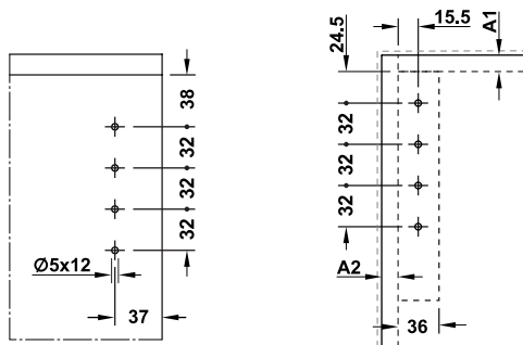
Drilling pattern for cabinet ระยะเจาะสำหรับตู้
